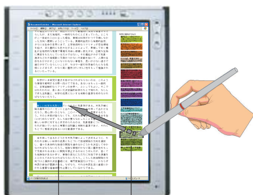
図 2 提案した Overview+Detail ドキュメントインタフェース Fig.2 Proposed Overview+Detail document interface.
